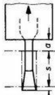
Fig. 12 Longueur d'outil
