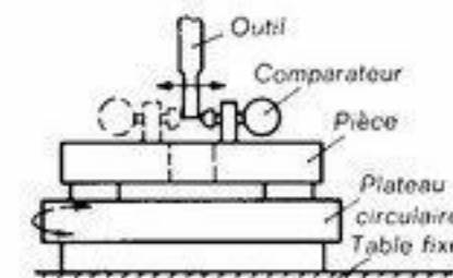
Fig. 15 Aligner l'outil sur l'alésage de la pièce
