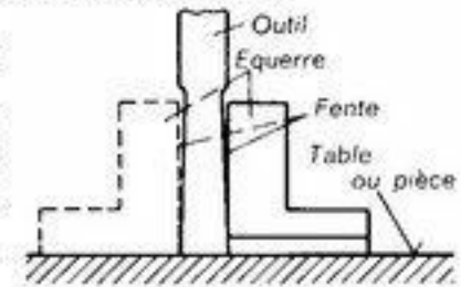
Fig. 14 Ajuster verticalement l'outil
