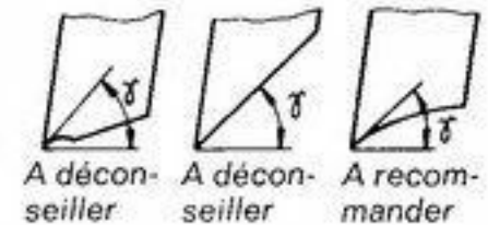
Fig. 11 Faces d'attaque pour des angles \delta importants
