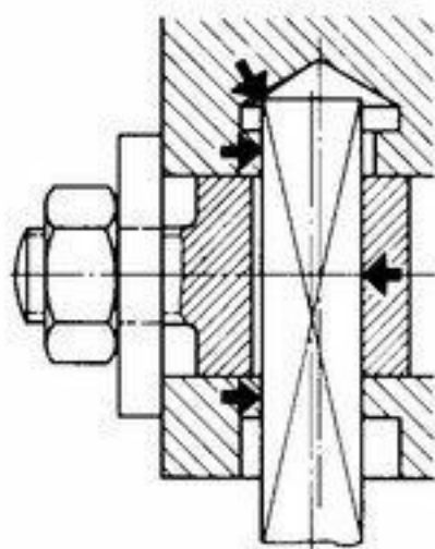
Fig. 13 Outil correctement serré
